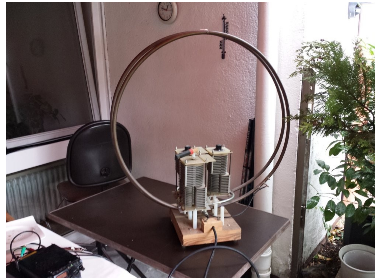
Magnetantenne
